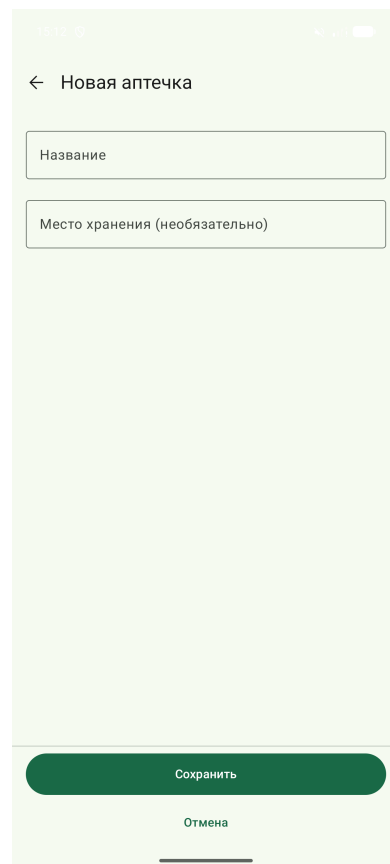
Рис. 2. Заведение аптечки
