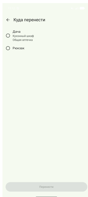
Рис. 7. Перенос упаковки
