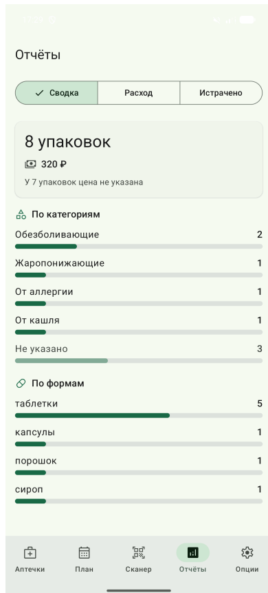
Рис. 22. Сводная статистика
