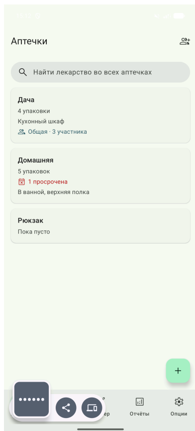
Рис. 1. Список аптечек
