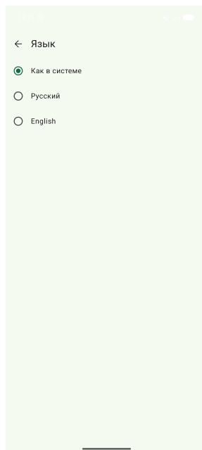
Рис. 36. Выбор языка
