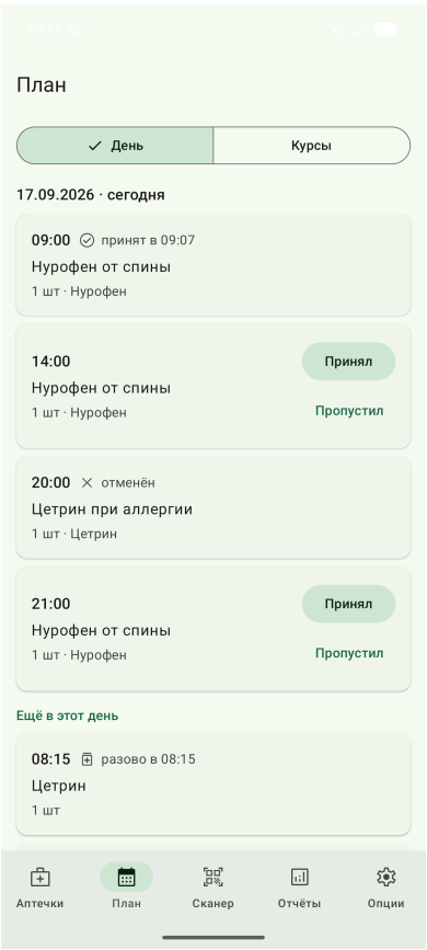
Рис. 15. План дня
