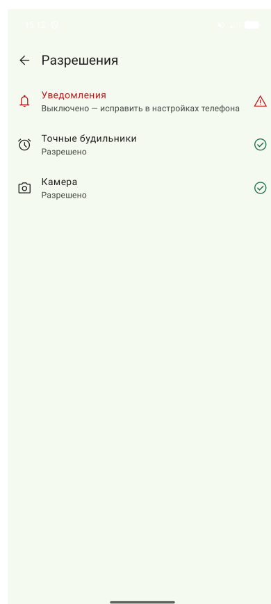
Рис. 35. Состояние разрешений
